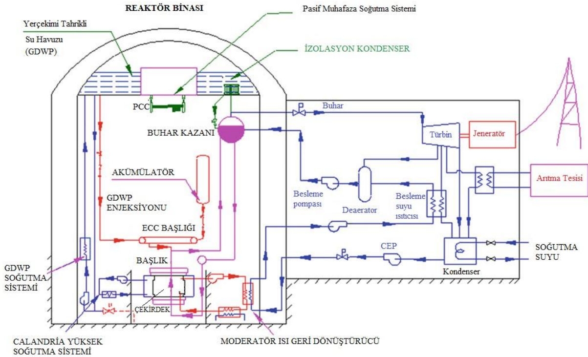
Şekil 2. Genel AHWR görünümü (Yemelyanov, 1969)
