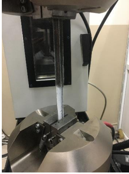
Şekil 3. Instron 8801 ile çekme deneyi.
