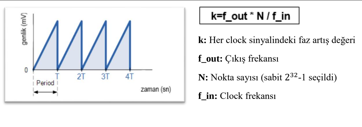
Şekil 3. Faz Register'in çalışma mantığı
