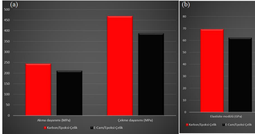
Şekil 6. Hibrid kompozitlerin mukavemet değerleri; (a) akma ve çekme dayanımları, (b) elastisite modülleri.
