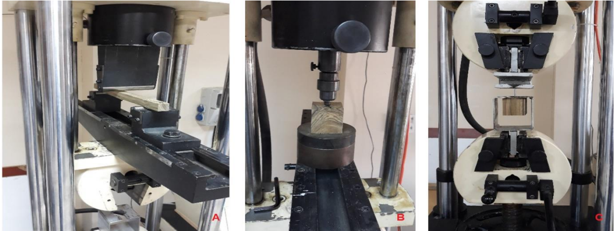
Şekil 4. Eğilme direnci deney düzeneği (A), Statik sertlik deney düzeneği (B), Vida tutma kapasitesi deney düzeneği (C).
