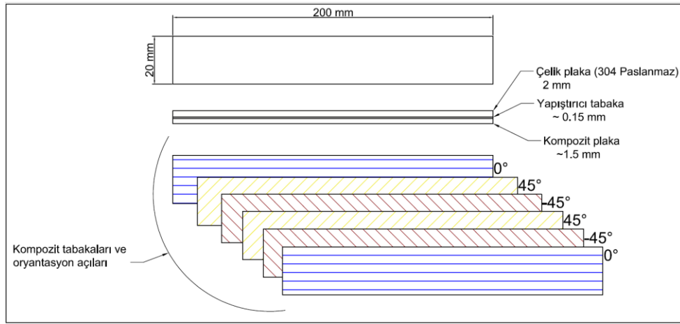
Şekil 2. Hibrid deney numunesi ölçüleri ve kompozit kısmın tabaka oryantasyon açıları.
