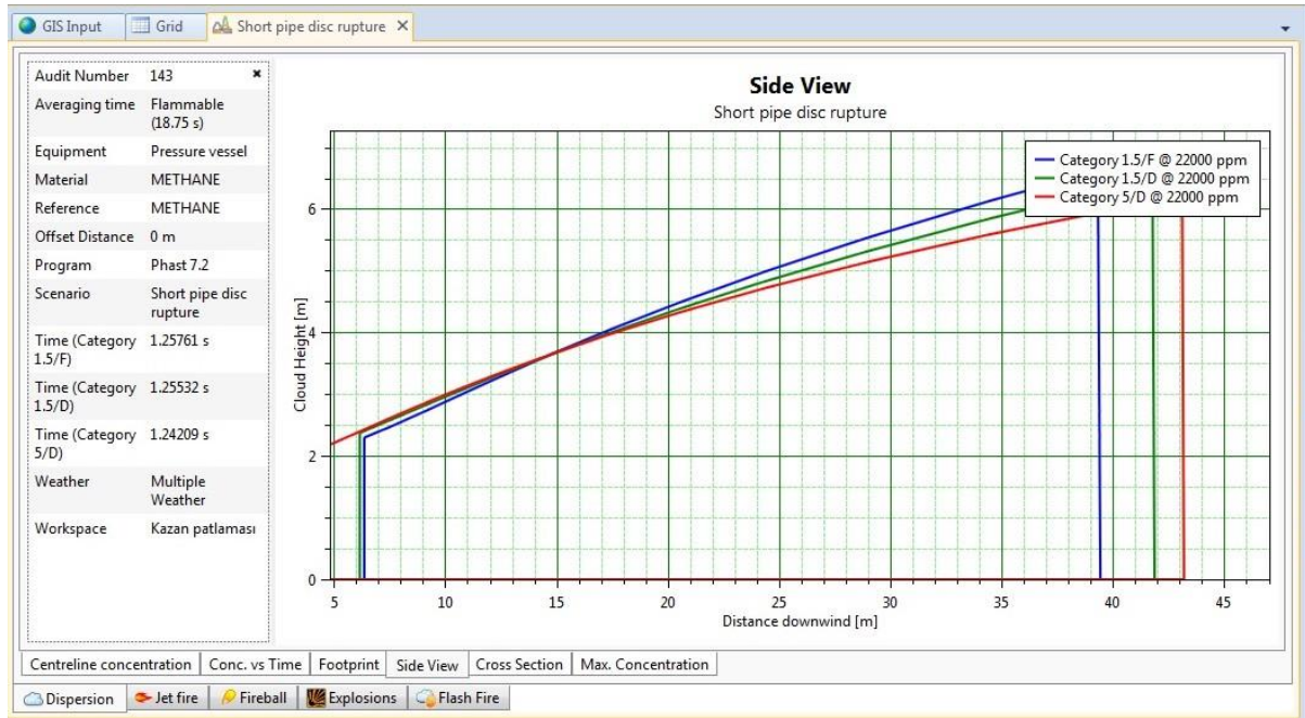
Şekil 6. Boru yırtılması (disc rupture) senaryosunda, yandan kesit görüntüsü
