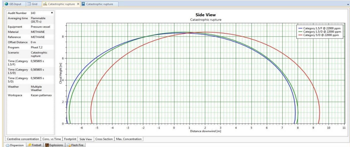
Şekil 5. Katastrofik yırtılma senaryosunda, yandan kesit görüntüsü
