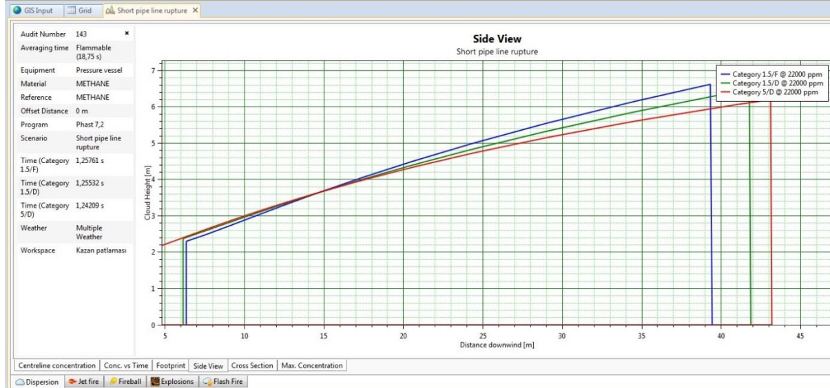
Şekil 8. Kısa boru yırtılması (line rupture) senaryosunda, yandan kesit görüntüsü
