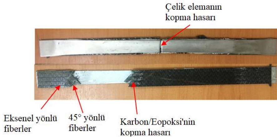
Şekil 4. Hasarlı hibrid numuneler.
