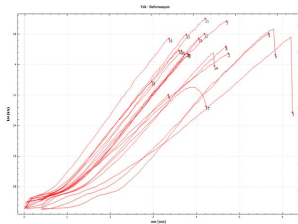
Vida tutma kapasitesi Enine yön(D)
