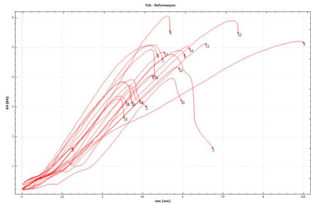
Vida tutma kapasitesi Teğet yön (B)
