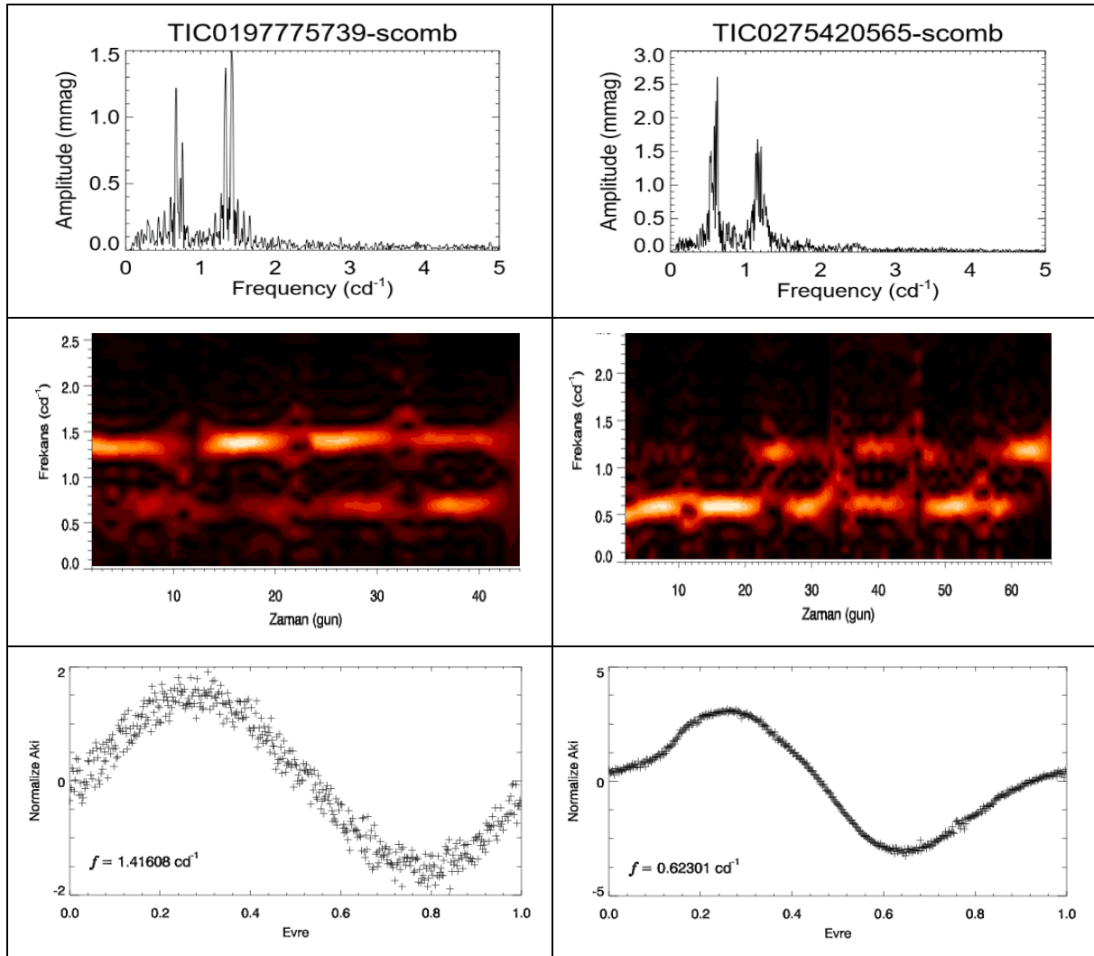
Şekil 2: Üst satır: TIC0197775739 ve TIC0275420565 yıldızları için LS yöntemi ile elde edilmiş periodogramları, orta satır: ışık eğrilerindeki frekans ve genliklerin zamana bağlı değişimlerini ve alt satır: Tablo 1’de verilen temel mod kullanılarak evrelendirilmiş ışık eğrilerini göstermektedir.
