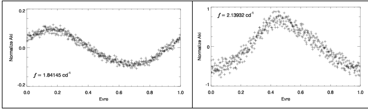
Şekil 1: Üst satır: TIC140214221 ve TIC173956099 yıldızları için LS yöntemi ile elde edilmiş periodogramları, orta satır: ışık eğrilerindeki frekans ve genliklerin zamana bağlı değişimlerini ve alt satır: Tablo 1’de verilen temel mod kullanılarak evrelendirilmiş ışık eğrilerini göstermektedir.
