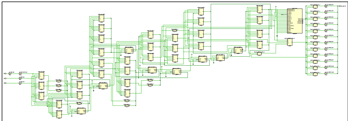
Şekil 5. Sistemin ikinci seviye RTL Şeması
