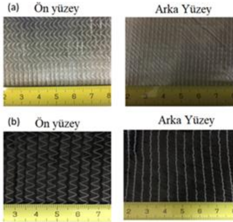
Şekil 1. Kompozit takviye kumaşları; (a) üç eksenli dikişli kıvrımsız E-cam kumaş, (b) üç eksenli dikişli kıvrımsız kumaş karbon.
