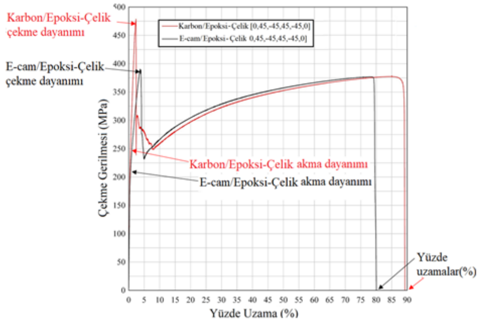
Şekil 5. Çekme-yüzde uzama eğrileri.
