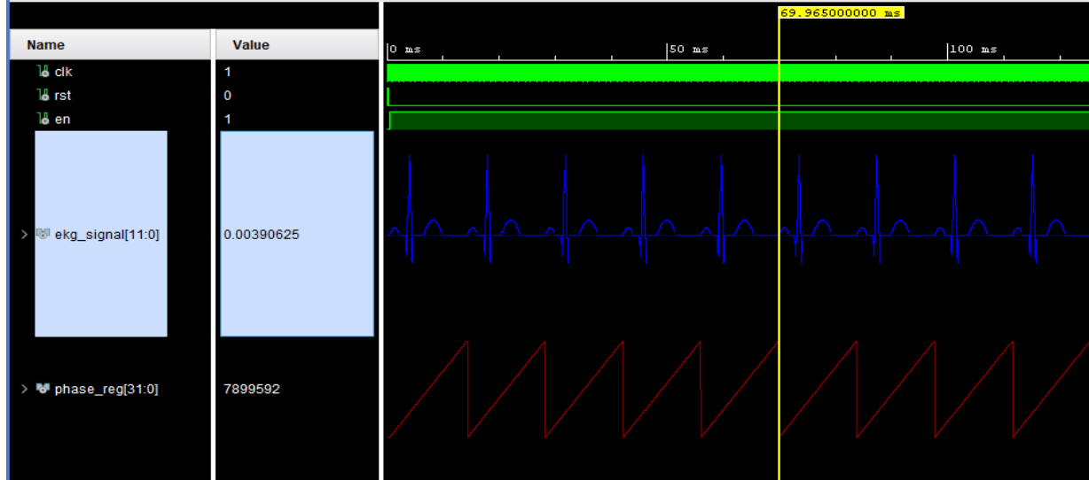
Şekil 6. Modellenen EKG sinyalinin faz regester'i ile Vivado simülasyonunda gözlemlenmesi
