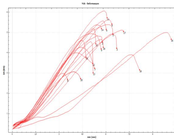
Vida tutma kapasitesi Radyal yön (C)
